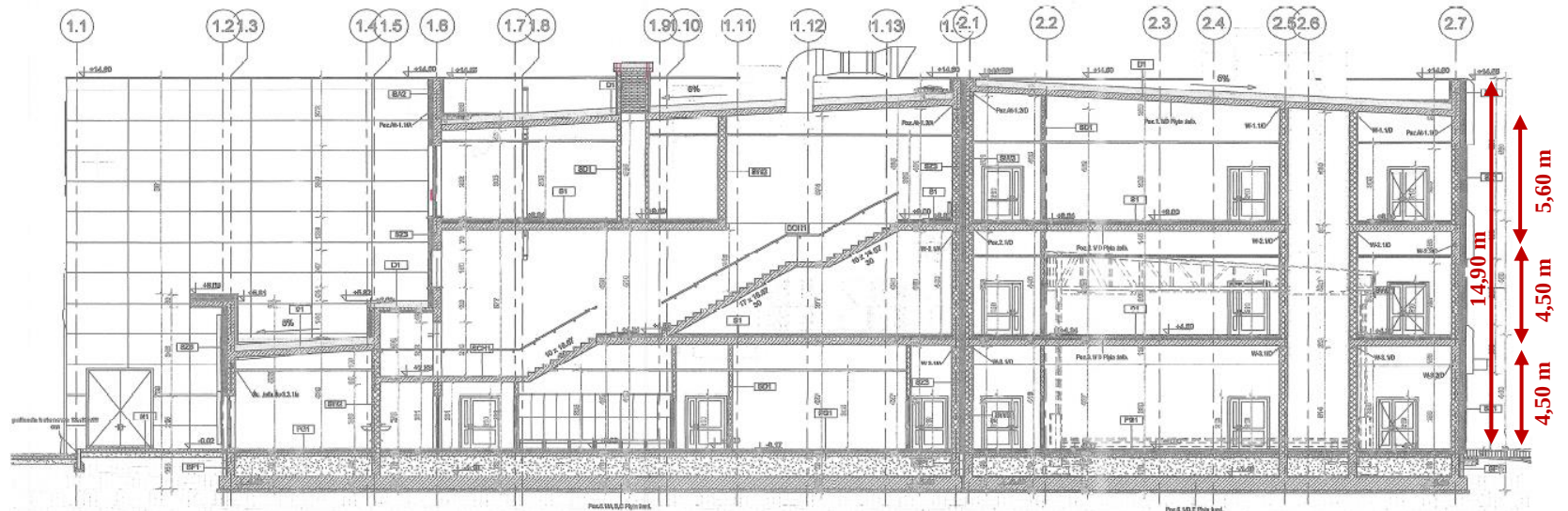
PRZESKÓJ D-D
