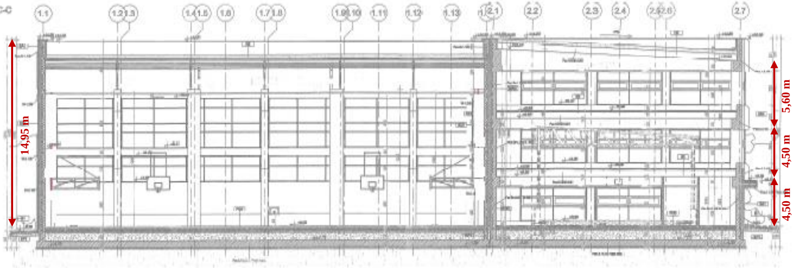
PRZESKÓJ D-D
