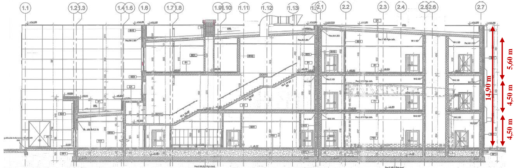
PRZEKRÓJ D-D
